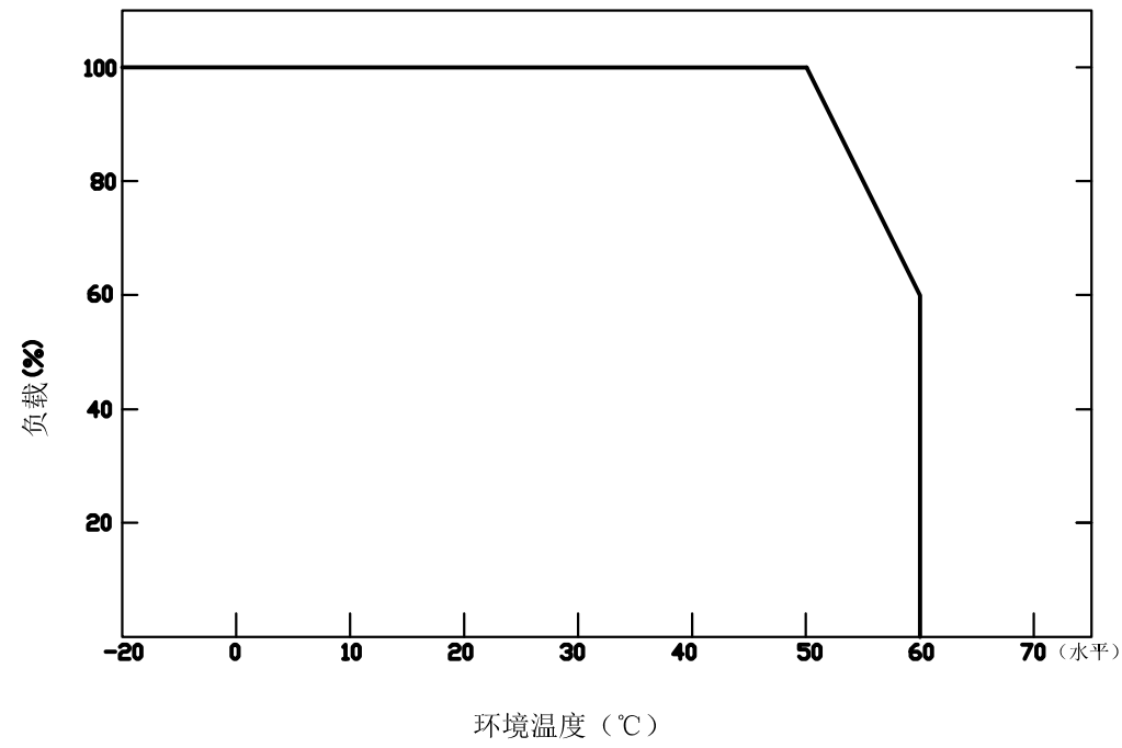
●负载减额曲线
