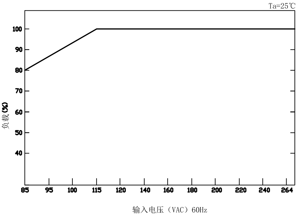
●静态特性曲线
